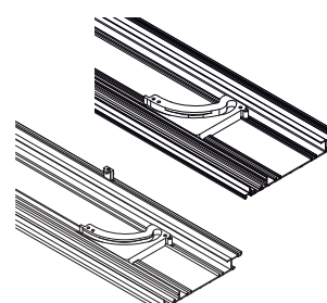
set de guías
