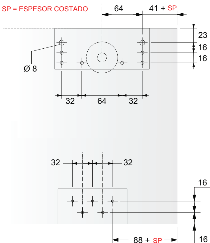
MONTAJE CARRIL INFERIOR Y SUPERIOR CLIP
