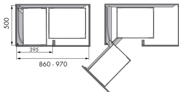
Apertura a izquierdas
