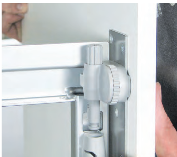
ClickFixx para MAGIC CORNER
