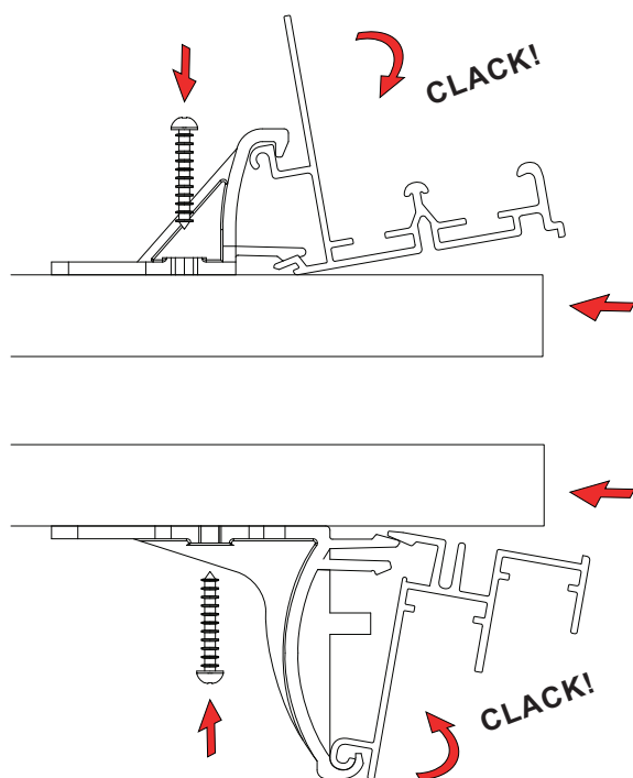
MONTAJE CARRIL INFERIOR Y SUPERIOR CLIP
