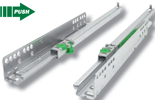
Detalle Bloqueo Antivuelco y Regulación en Altura Cajón
