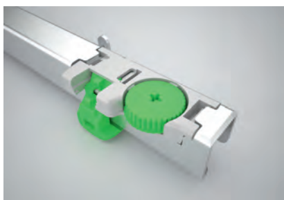
Detalle Bloqueo Antivuelco y Regulación en Altura Cajón
