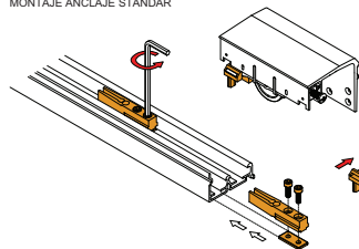
MONTAJE ANCLAJE STANDAR
