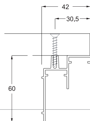
carril inferior atornillar
