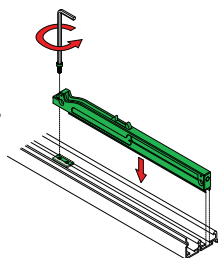
MONTAJE AMORTIGUADOR
