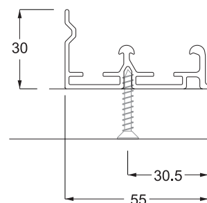
carril superior atornillar
