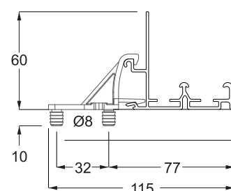
carril superior clip
