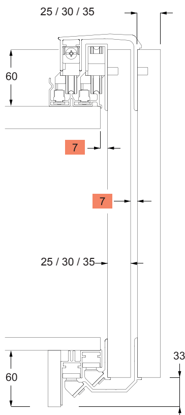
MONTAJE CARRIL INFERIOR Y SUPERIOR CLIP
